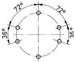
孔样式 4
